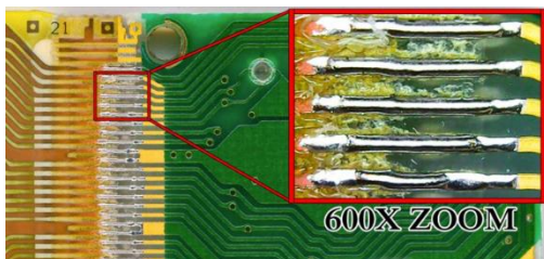
Abbildung 3 Verlöten eines Flachkabels mit dem Display
